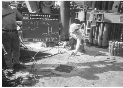
7" ケーシングパイプ挿入
