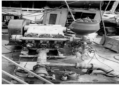
温泉工専用ポンプ・機械
