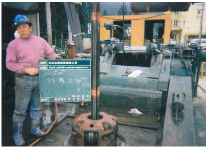
ケリーホール掘削
