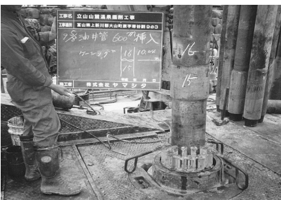
ケーシング 16-17
