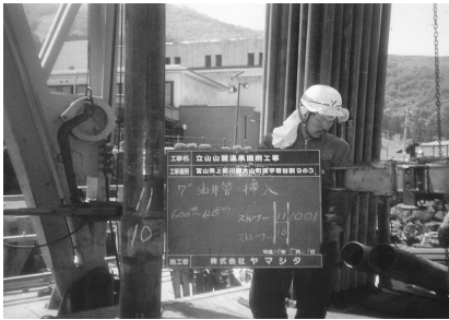
7" ストレーナー挿入 10-11
