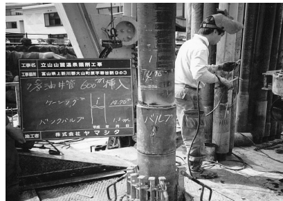
ケーシング 1
