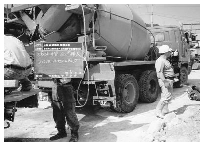
フルホールセメンチング
