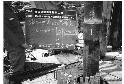
ケーシング 1-2
