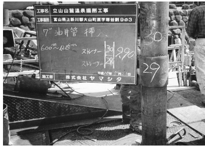
油井管 600m ケーシング 29-30
