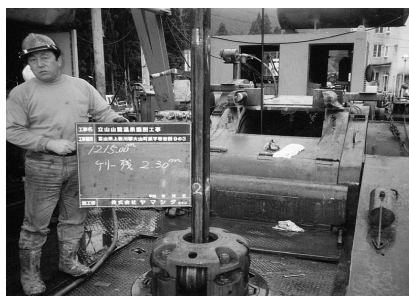
1,215m ケリー残 2.30m
